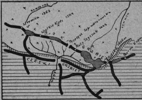
Geologiczny szkic Karkonoszy.
