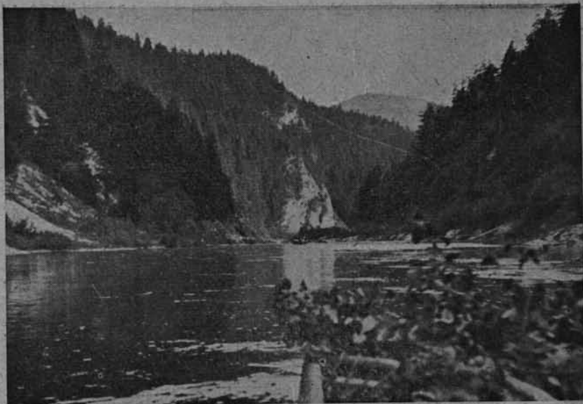
Pieniny: Podłużne odcinki przełomu dunajcowego są nieco łagodniejsze.
