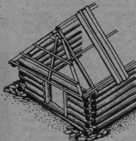
Szalas w dolnej partii hali Na Stołach. Powyżej na prawo: szczegół więzara dachowego. Obok: widok aksonometryczny.
