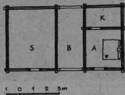
Plan szalasu na hali Jaworzynka. A — izba, B — boisko, K — komora, S — stajnia, W — watrzyśko.
